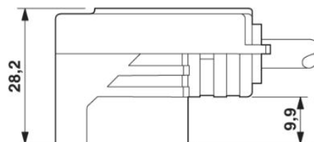
Ventilstecker, Bauform B, Seitenansicht
