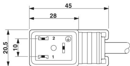
Ventilstecker, Bauform B
