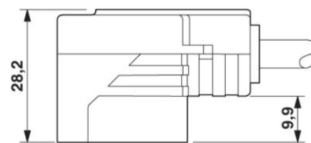
Ventilstecker, Bauform A, Seitenansicht
