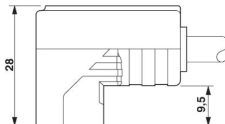
Ventilstecker, Bauform C, Seitenansicht
