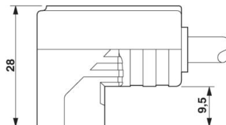
Ventilstecker, Bauform CI, Seitenansicht
