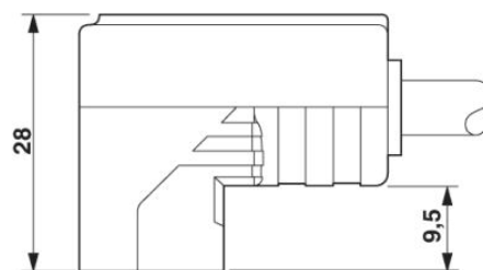
Ventilstecker, Bauform CI, Seitenansicht
