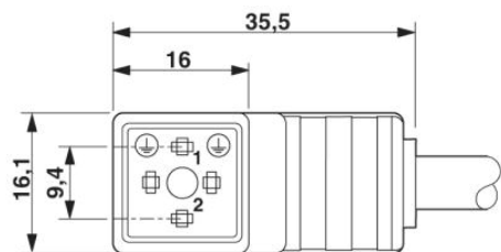
Ventilstecker, Bauform CI
