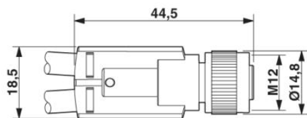
Stecker M12 x 1, gerade, geschirmt
