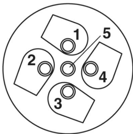
Kabelanschlusssseite M12 (Schraubanschluss)
