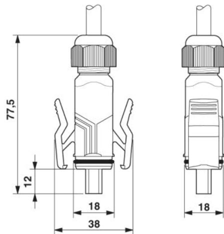
USB-Steckverbinder, Typ B, IP67
