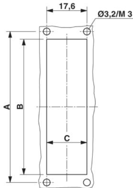
Montageausschnitt: VS-25-A...
