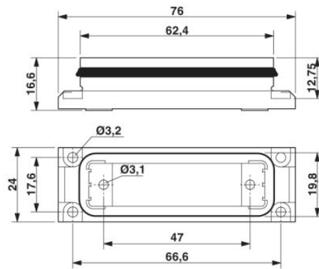
D-SUB Anbaurahmen
