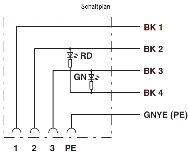
Kontaktbelegung des Ventilsteckers
