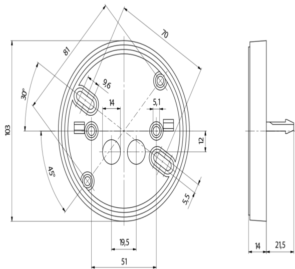
Bemaßung 92161
