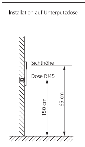
Installation mit Patchkabel
