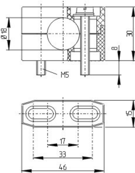
Maßzeichnung (Grundgerät)
