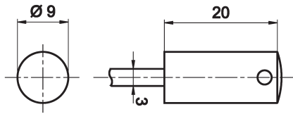
Massbild
