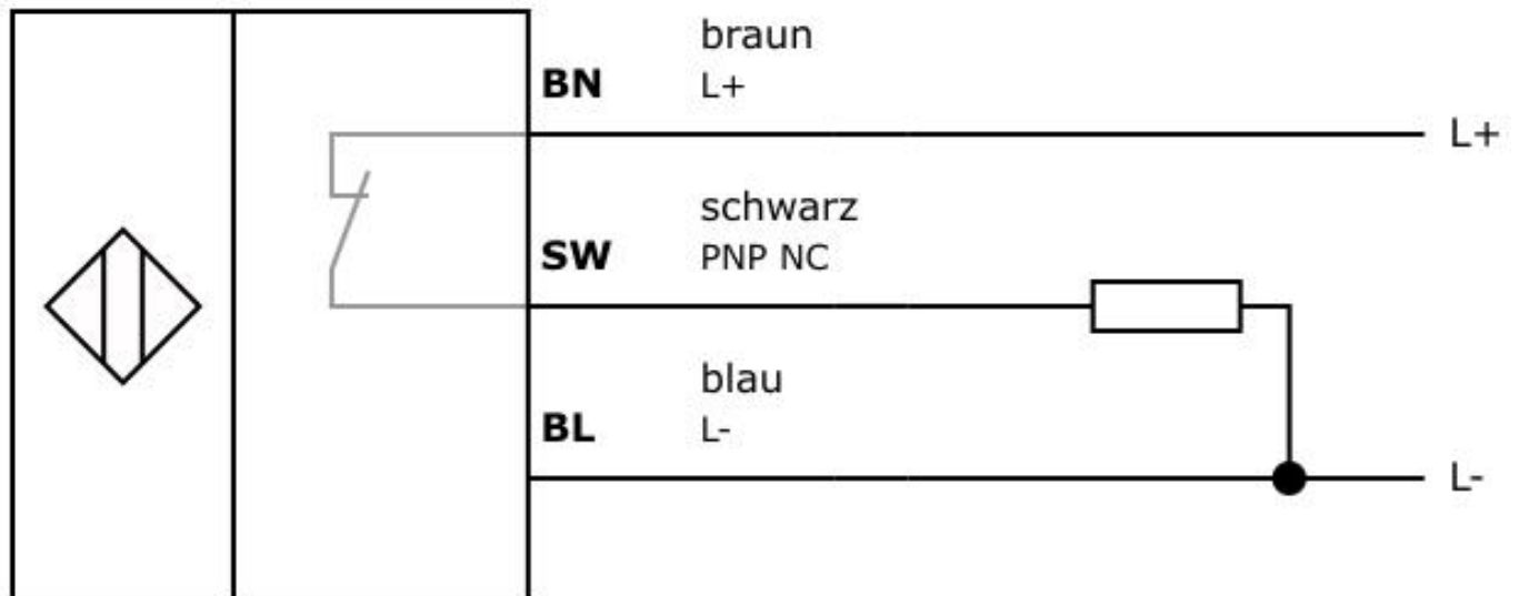
Anschlussbild
