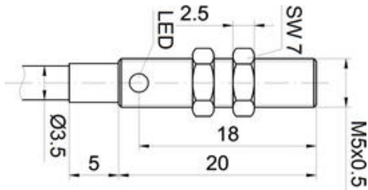
Massbild
