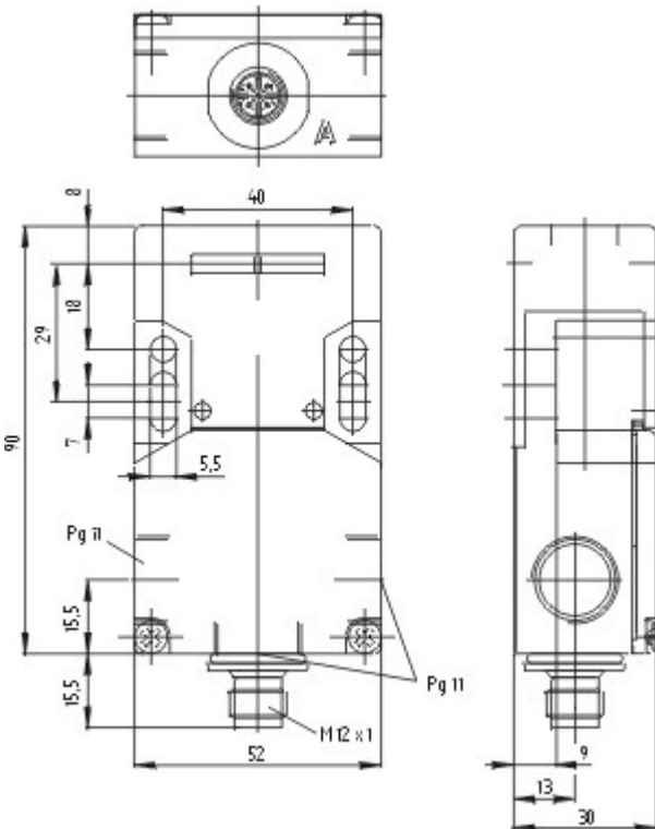
Maßzeichnung (Grundgerät)
