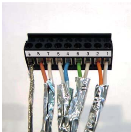
Afb. 12: Aansluitblok
