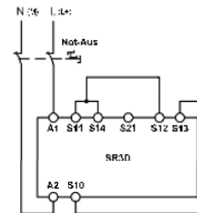
Abb. 8: Einkanalige Not-Halt-Schaltung ohne Fehlerüberwachung des Not-Halt-Tasters und der Zuleitungen. (Kategorie 1, bis PL c / SIL 1)
