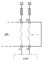
Abb. 16: Anschluss der Spannungsversorgung an den Klemmen A1 und A2. (Versorgungsspannung entspre- chend techn. Daten)
