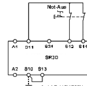
Abb. 4: Zweikanalige Not-Halt-Schaltung mit Querschluss- und Erdschluss- Überwachung (Kategorie 4, bis PL e / SIL 3)
