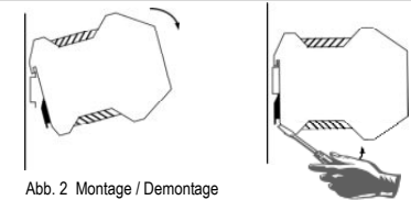
Abb. 2 Montage / Demontage
