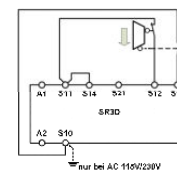
Abb. 6: Einkanalige Not-Halt-Schaltung mit Erdschluss-Überwachung. (Kategorie 1, bis PL c / SIL 1)
