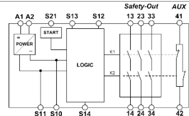
Abb. 1 Blockschaltbild SR3D
