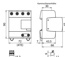
Maßbild DV M2 TT 255 FM
