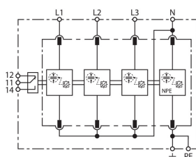
Prinzipialschaltbild DV M2 TT 255 FM
