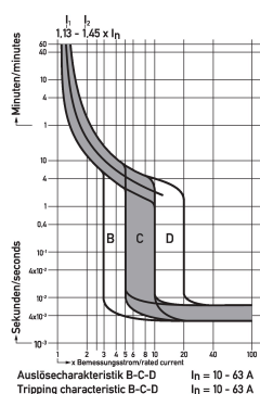
Diagramme Leitungsschutzschalter DLS 6i D10-1
