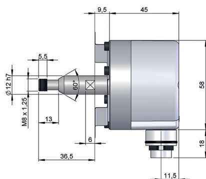
Maßzeichnung Vollwelle Typ 1, Drehmomentstütze Typ 4, Anschluss 2
