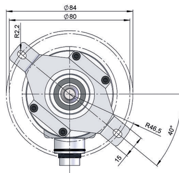
Maßzeichnung Vollwelle Typ 1, Drehmomentstütze Typ 4, Anschluss 2
