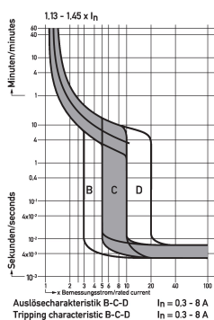
Diagramme Leitungsschutzschalter DLS 6i B1-3+N
