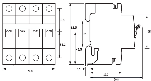
Maßzeichnung Leitungsschutzschalter DLS 6h B6-3+N
