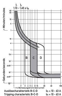
Diagramme Leitungsschutzschalter DLS 6h C20-2
