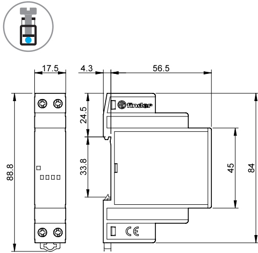
Typ 78.36 Schraubklemmen
