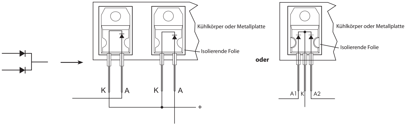
Diode für Typen 78.25, 78.36, 78.50, 78.60, 78.61
