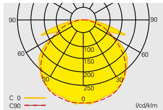
Lichtverteilungskurve SV EURO 4 LED mit klarer Haube
