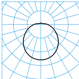
Mondia G2 WD1 LED1000-840 ETDD TX050105
