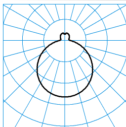
74R WD1 LED1000-840 TX054545
