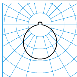
74R WD2 LED2000-840 TX054269
