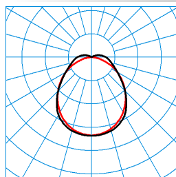
OleveonF 1200 4000-840 PC+LLWC LV TX056118
