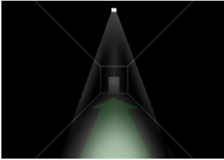
Fluchtwegausleuchtung für 1 lux Asymmetrisch 75°-75° Neigungswinkel
