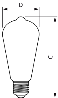
ST64 230V 60W 806lm 2700-2200K E27 D CL
