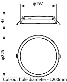
DN065B G3 LDNR LED20/CCT 19.5W D200 RD
