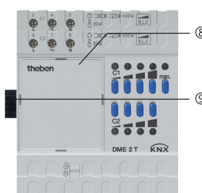
DME 2 T KNX (Erweiterungsmodul)
