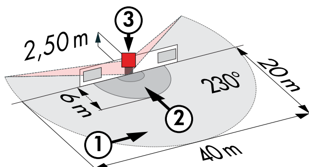
Reichweitendiagramm
