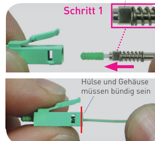
Abb.: LC/APC Steckergehäuse anbringen
