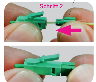
Abb.: Verriegelung anbringen
