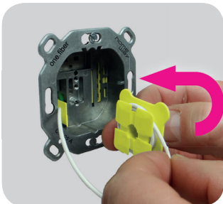
Abb.: Glasfaserkabel auf Spule wickeln
