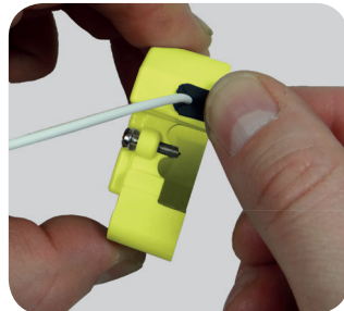
Abb.: Klemmgummi in Schutzdeckel bringen
