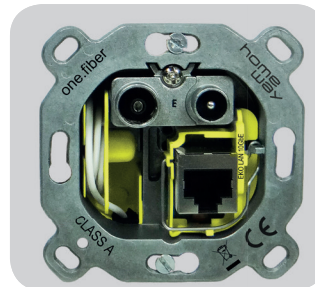
Abb.: Dose mit Speicherspule und Modulen
