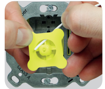
Abb.: Einführen Kabel in Speicherspule
