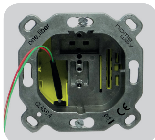
Abb.: Dose in der Wand
