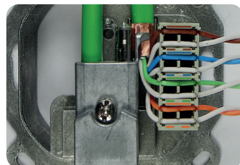
Abb.: Adern auflegen
