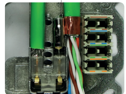
Abb.: Kabel auflegen
