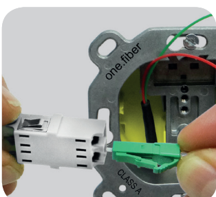
Abb.: LC/APC-Stecker in Kupplung stecken
