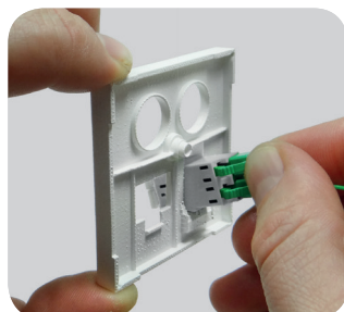
Abb.: Kupplung in die Zentralplatte stecken
