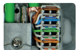
Abb.: Überstehende Adern abgeschnitten
