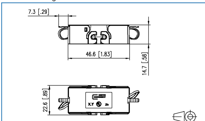
Masszeichnung
