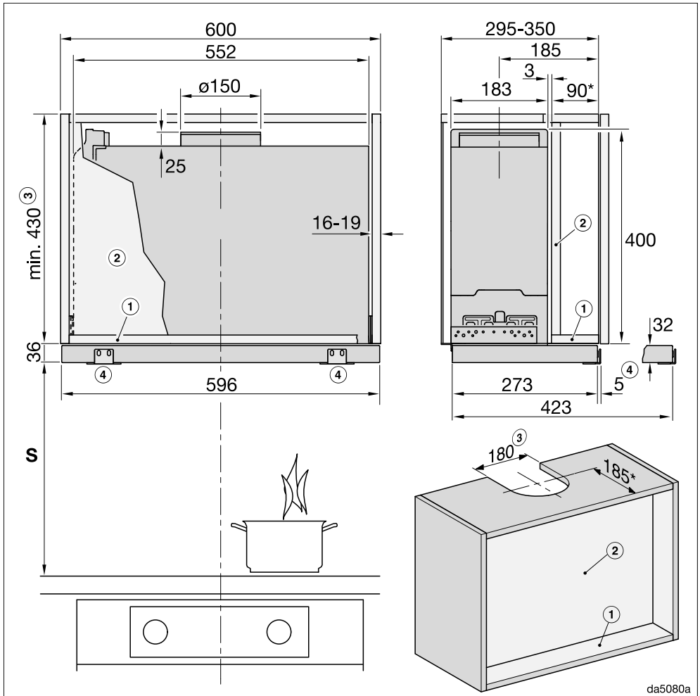
Bild 1: DAS 4620 in einem 600 mm breitem Schrank.
