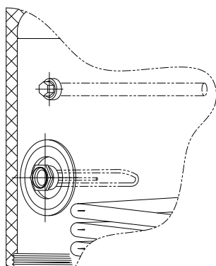
Fig. 8.1: Anode de la résistance électrique
