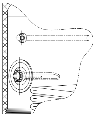
Abb. 8.1: Anode Elektroheizung
