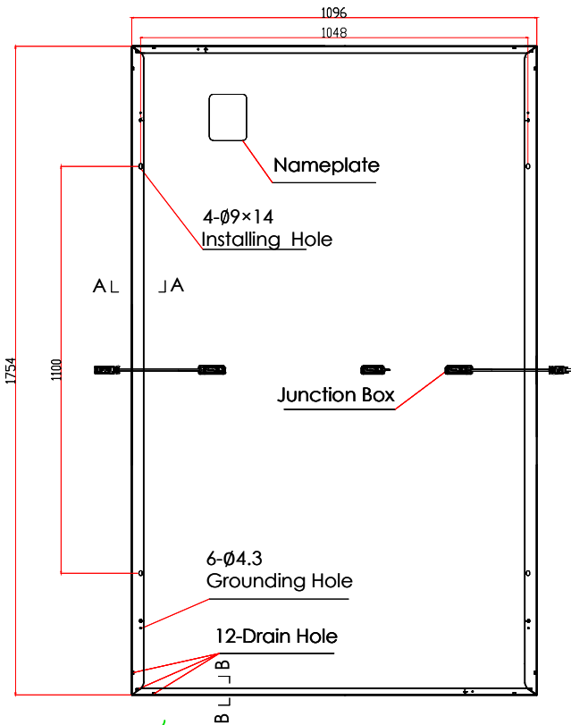
后视图
