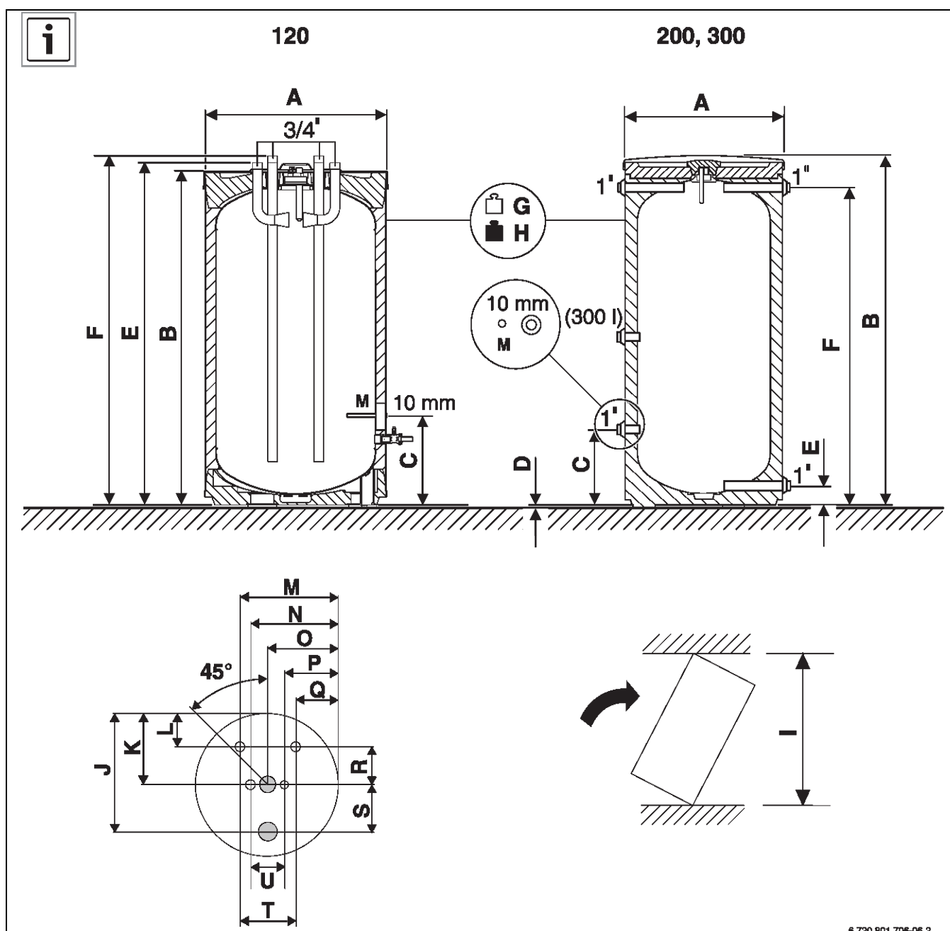
Bild 207 Abmessungen BH ...-5
