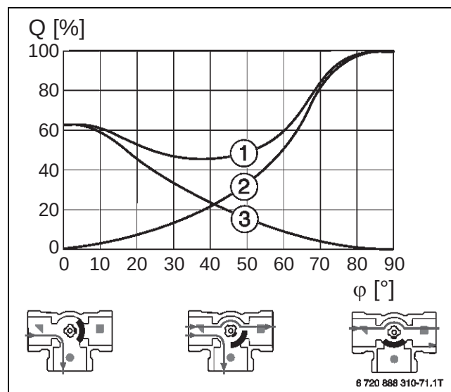
Bild 234 Mischerkennlinie
