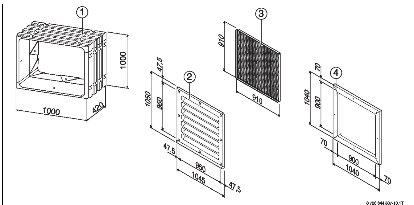
Bild 42 Wanddurchführung, Wetter-/Regenschutzgitter, Maschendrahtgitter und Verblendraahmen des Systems Luftkanal (Maße in mm)
