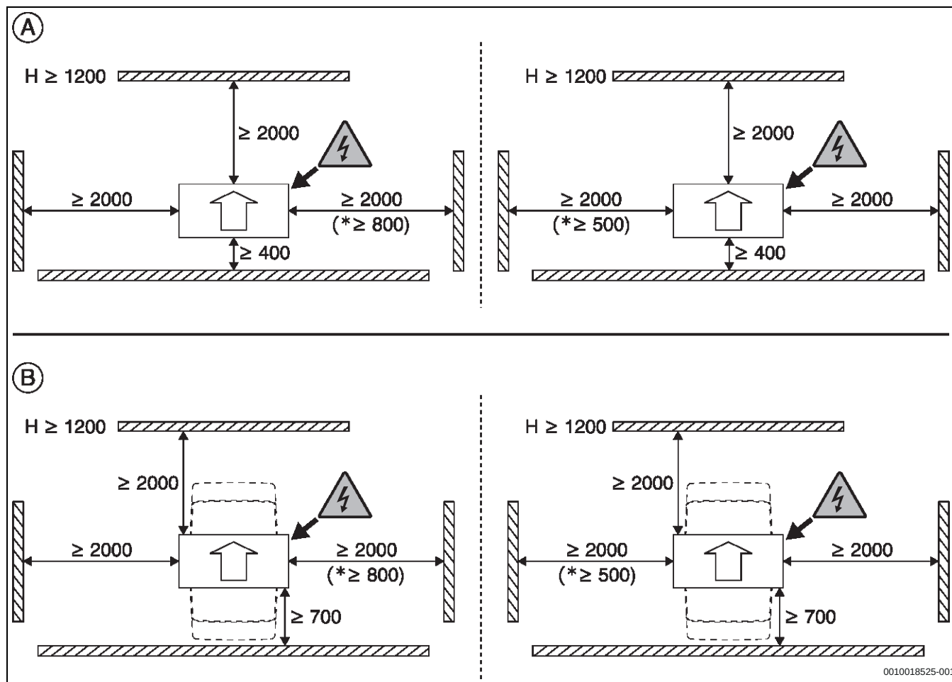
Bild 49 Mindestabstände CS7001iAW/CS7400iAW (Maße in mm)
