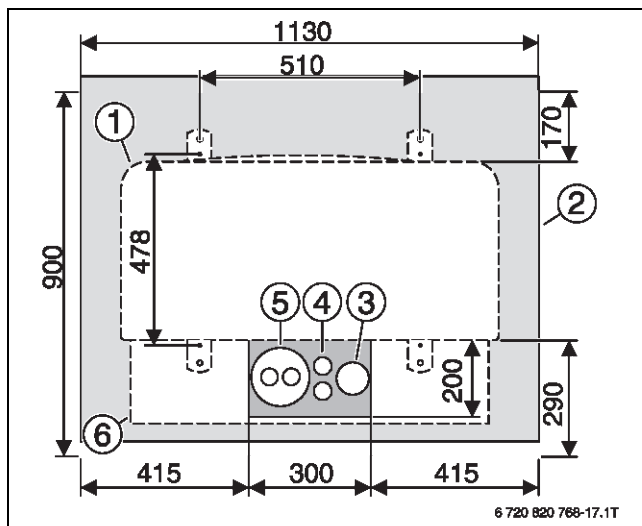
Bild 54 Abmessungen der Fundamentplatte und der Ausparung für die Rohre (CS7001iAW 5 OR...-S/CS7001iAW 7 OR...-S/CS7001iAW 9 OR...-S)
