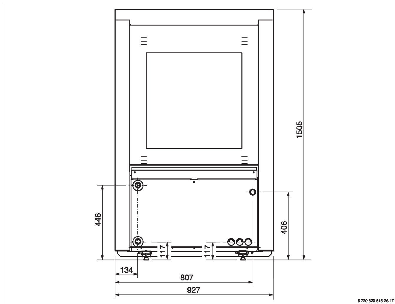
Bild 78 Abmessungen und Anschlüsse CS7000iAW 7 IR...-S/CS7000iAW 9 IR...-S, Rückseite (Maße in mm)
