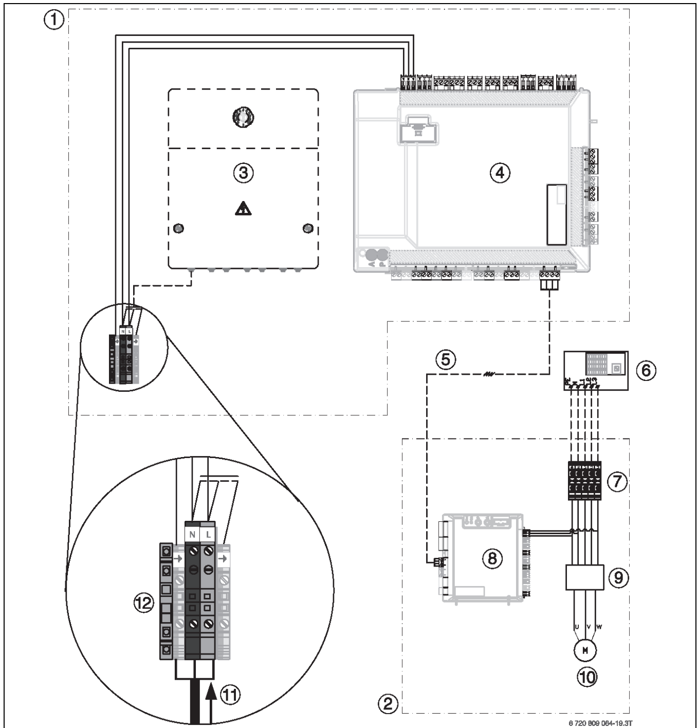
Bild 156 Wärmepumpen-Inneneinheit mit externem Zuheizter – Überblick
