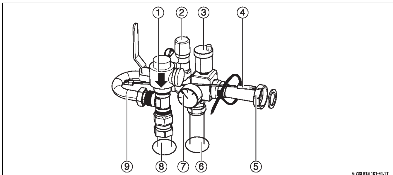
Bild 114 Montierte Sicherheitsgruppe
