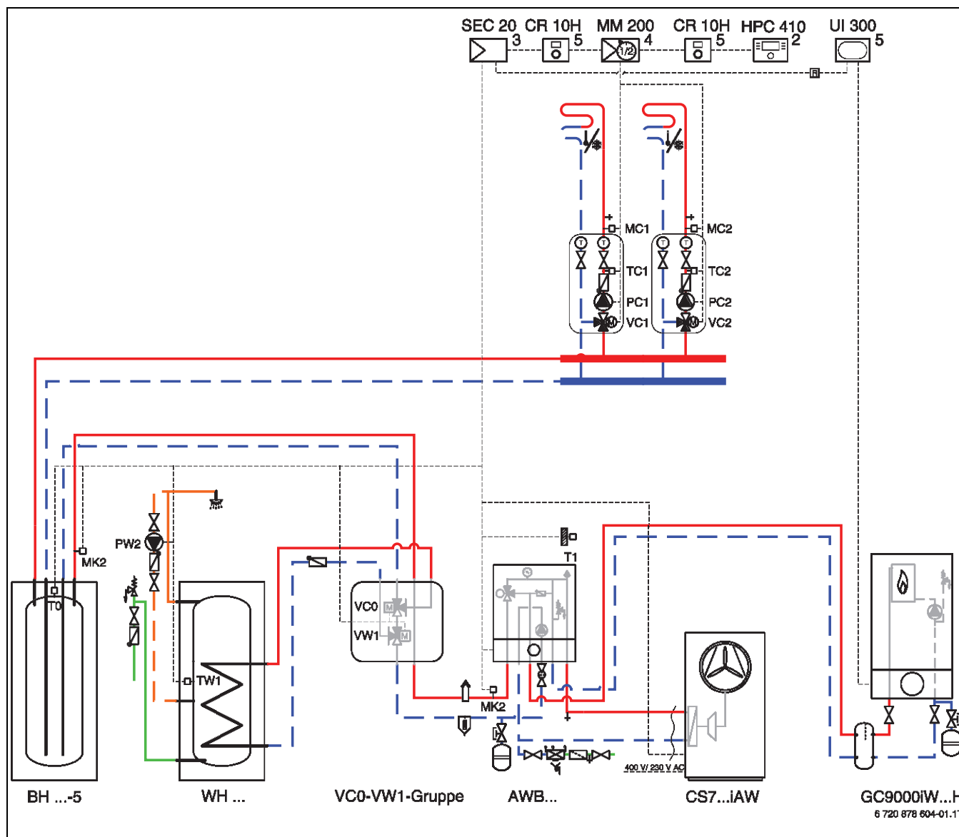
Bild 17 Anlagenschema mit Regelung (unverbindliche Prinzipsdarstellung)
