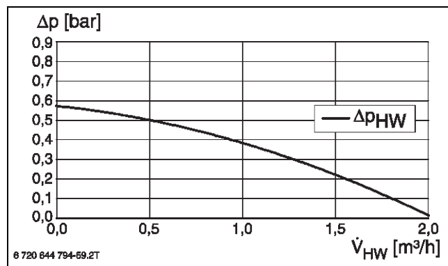
Bild 84 Restförderdruck CS7001iAW 5 OR...-S
