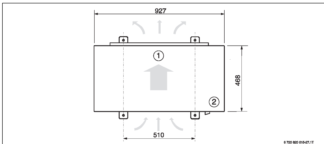
Bild 79 Abmessungen CS7000iAW 7 IR...-S/CS7000iAW 9 IR...-S, Draufsicht (Maße in mm)
