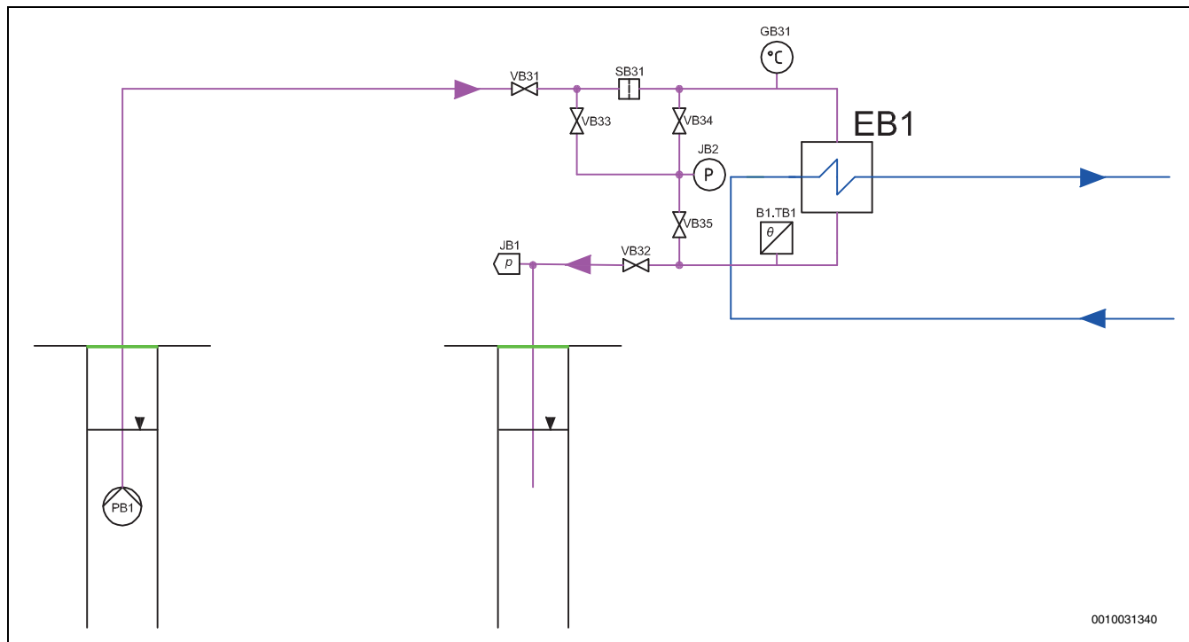
Bild 54 Grundwassersystem
