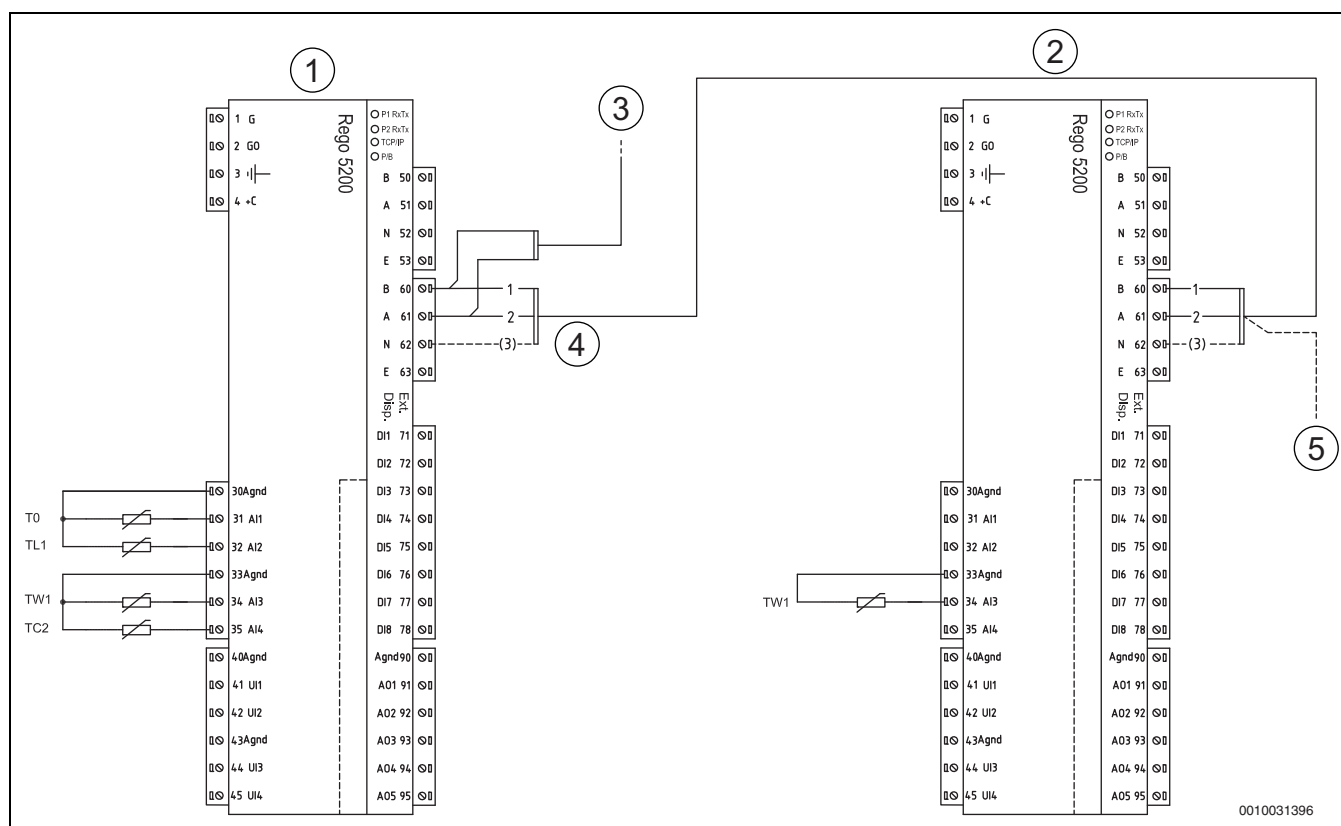
Bild 49 Schaltplan Kaskadenschaltung
