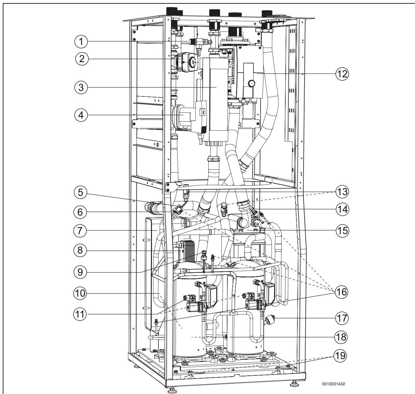
Bild 2 Produktübersicht 22–28 kW
