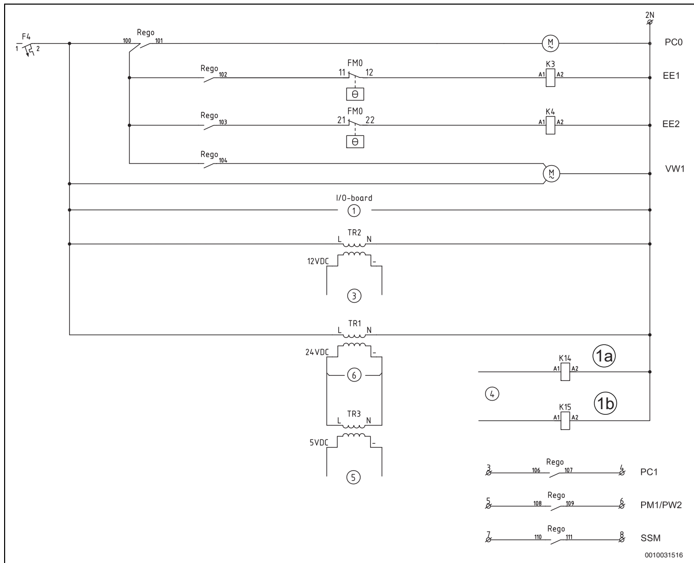
Bild 35 Schaltplan 22–28 kW
