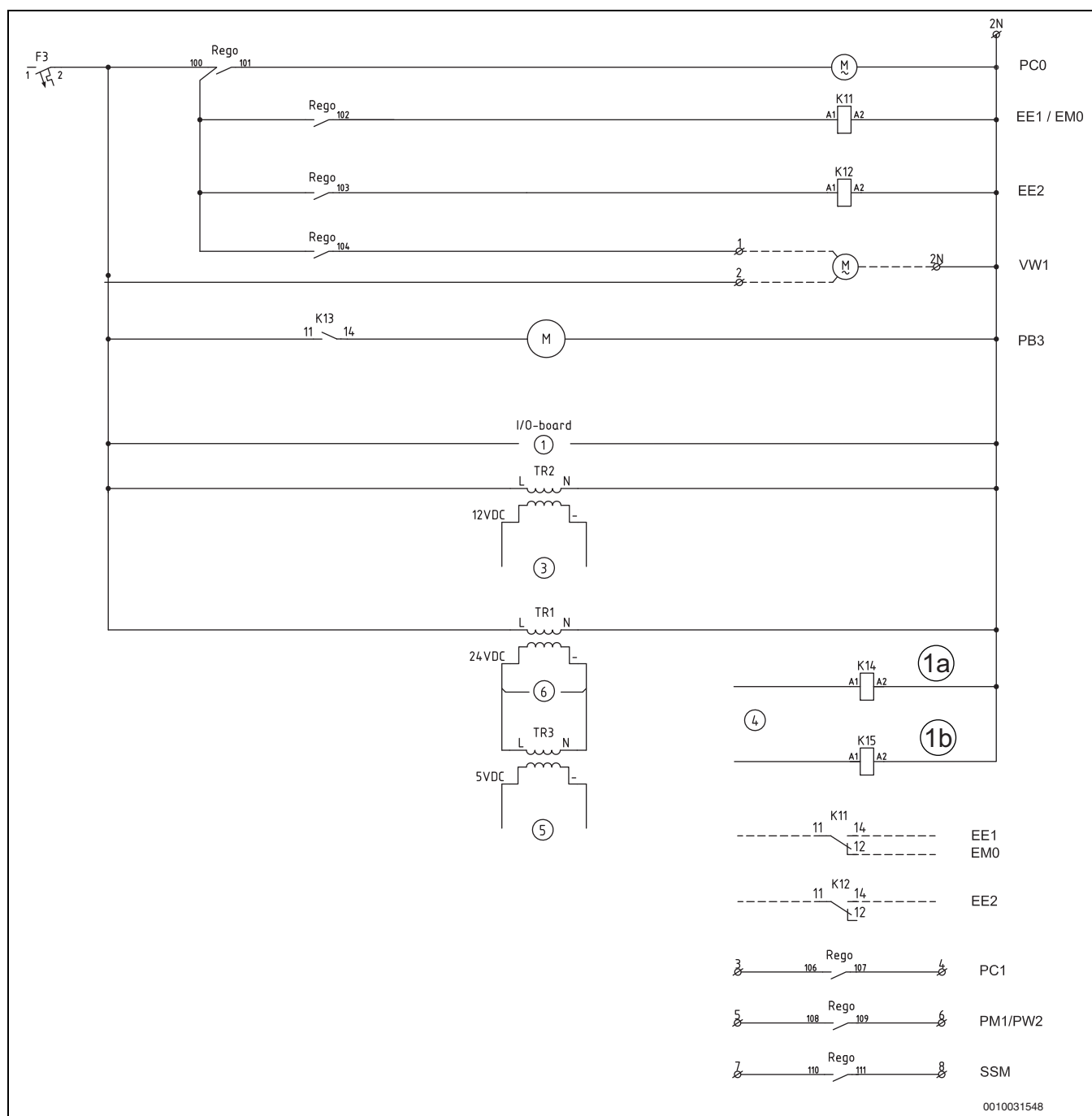
Bild 47 Schaltplan 38–48 kW
