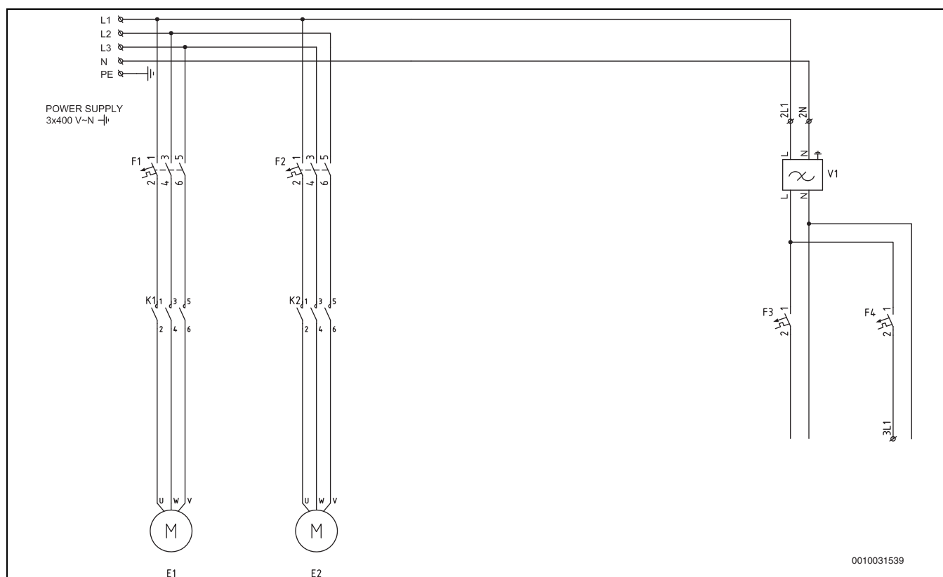
Bild 41 Betriebsschaltplan mit Schütz (38–48 kW)
