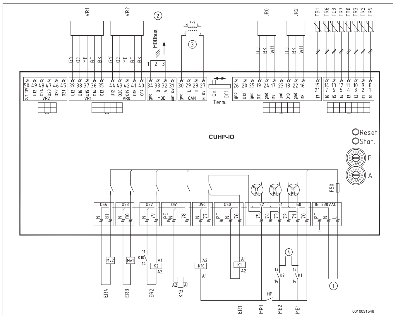
Bild 45 Schaltplan mit Schütz (38–48 kW)
