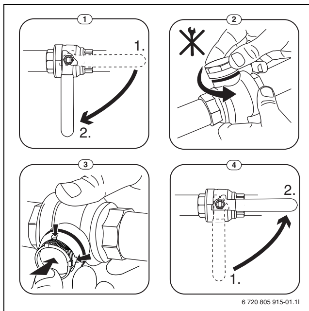
Bild 22 Siebreinigung
