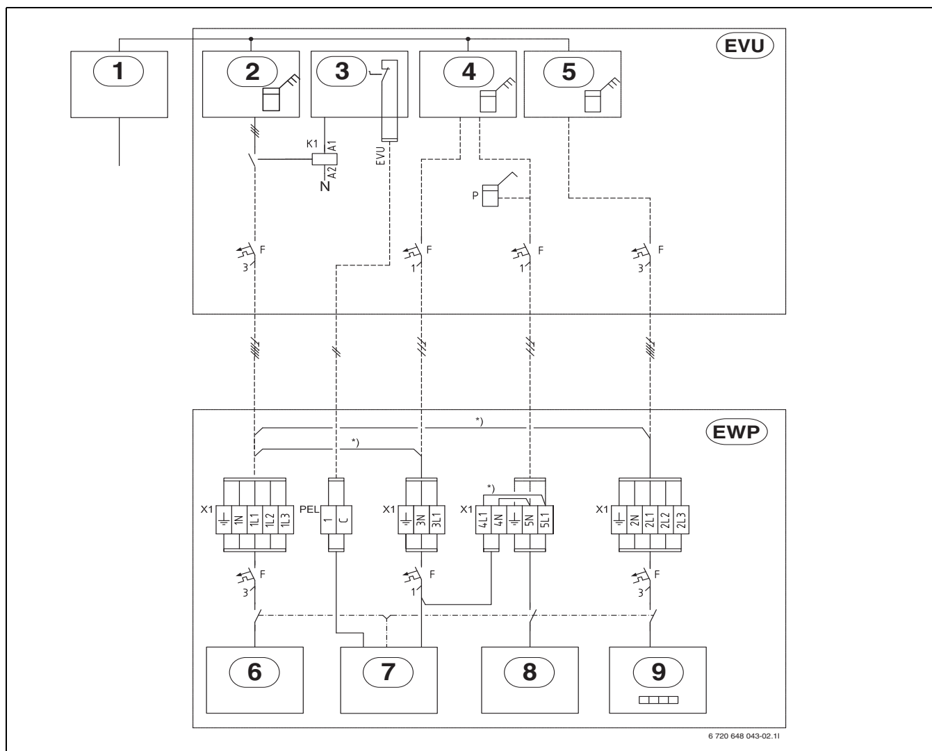
Bild 30 Anschlussübersicht Elektroschaltschrank - Wärmepumpe
