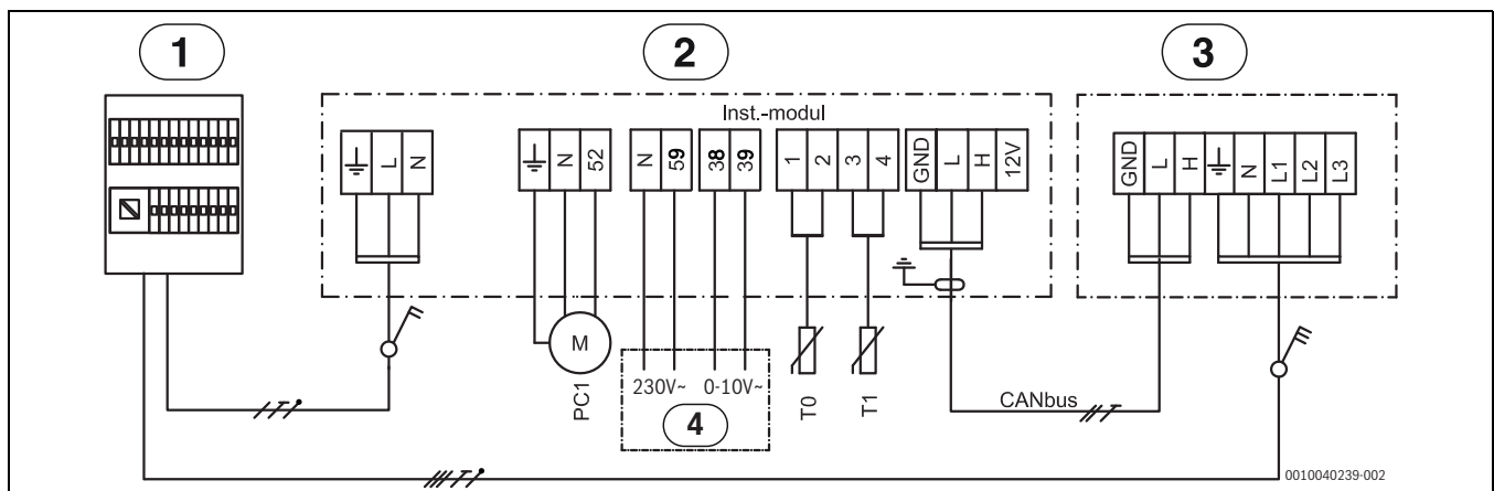
Bild 43 Schaltplan
