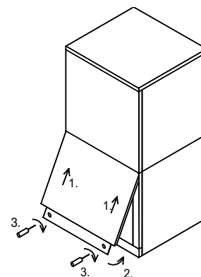
Zamykanie pokrywy
