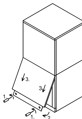
Otwieranie pokrywy
