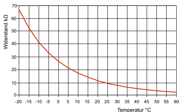
Abb. 9.1: Fühlerkennlinie NTC-10
