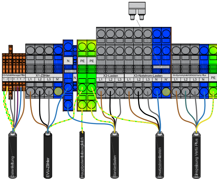
"Große" Steckbrücke X3 - N/N'
