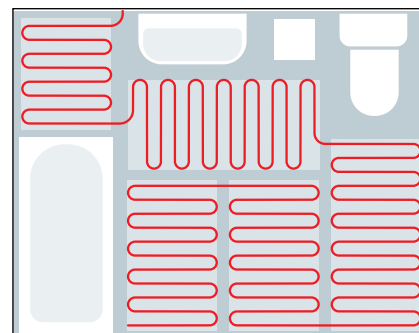
Verlegebeispiel
