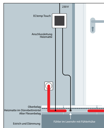
Installationsbeispiel
