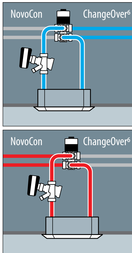
Heiz- und Kühldecken mit ChangeOver 6 -Umschaltung
