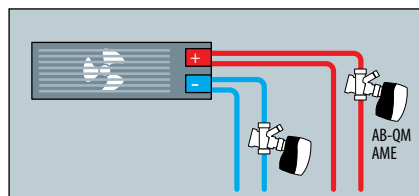
Lüftungs- und Klimagerät (air handling unit)
