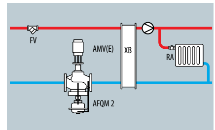
Indirekt angeschlossene Hausanlagen
