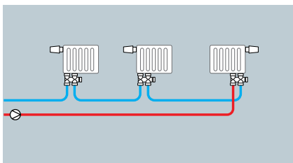
Ventileinsatz in Einrohranlage
