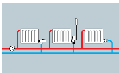
Einbau als Austauschventil für installierte Rücklauftemperaturbegrenzer
