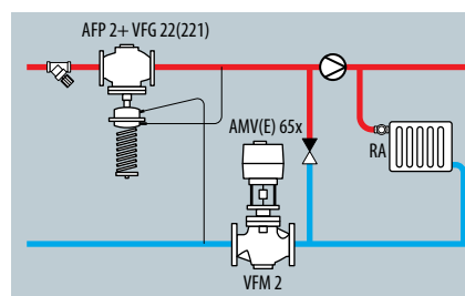
Direkt angeschlossene Hausanlagen
