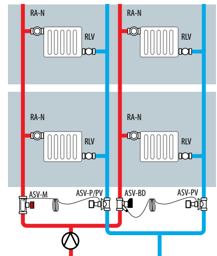
Anwendungsbeispiel
