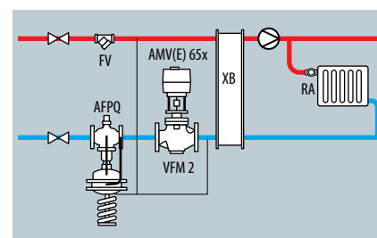
Indirekt angeschlossene Hausanlagen
