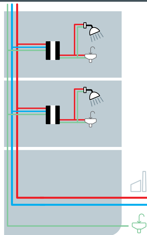
Dezentrale Trinkwassererwärmung
