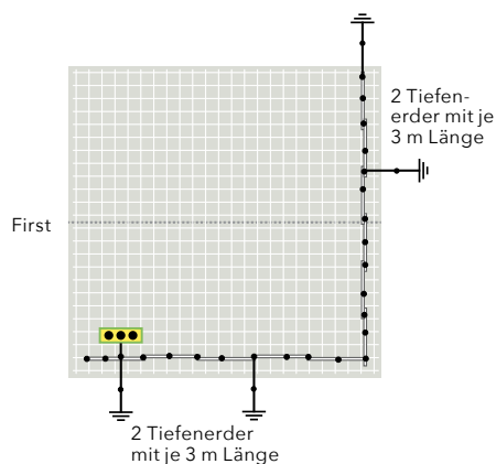
Variante 2: 4 x 3 m Tieferender
