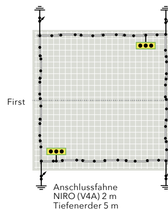
Variante 3: 4 x 5 m Tieferender (2 Erdungssets)
