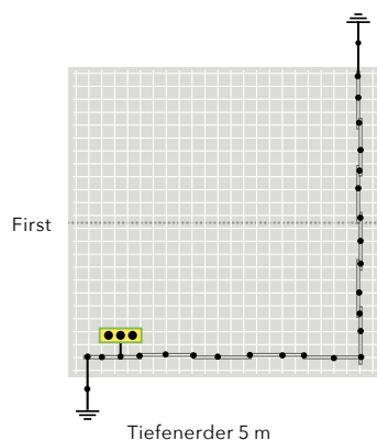
Variante 1: 2 x 5 m Tieferender
