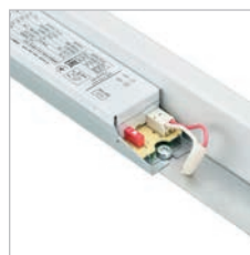
Lichtträger mit einstellbarem Lichtstrom (Dip-Switch). Ab Werk auf den höheren Lichtstrom eingestellt.
